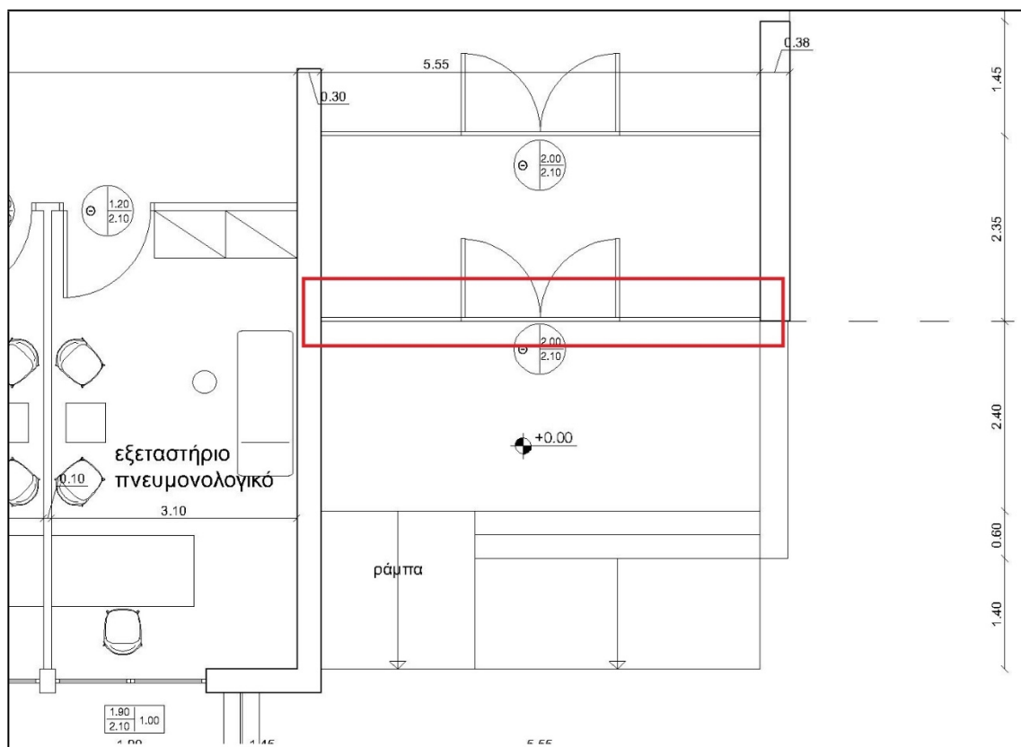
Σχέδιο 2: Απόσπασμα εισόδου εξωτερικών ιατρείων
